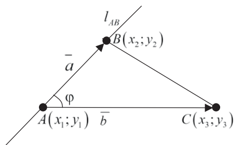
Рис. 1. К задаче о трех точках на плоскости
