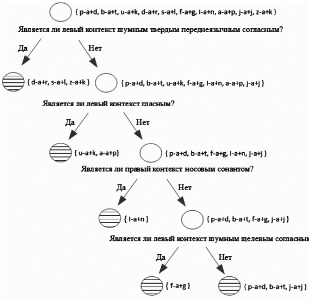
Рис. 1. Пример дерева регрессии для фонемы «а»
