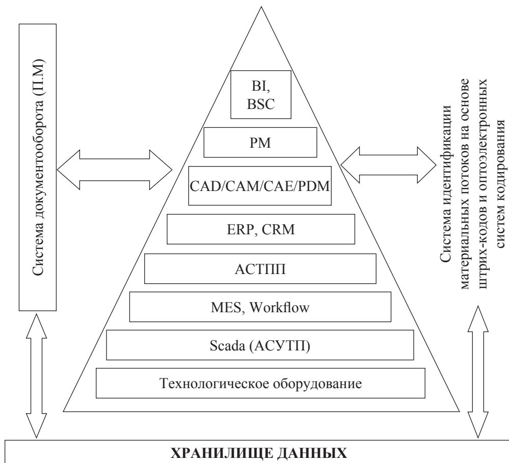
Рис. 1. Типовая структура корпоративной информационно-управляющей системы промышленного предприятия
